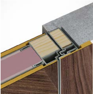
Короб реверсивного открывания RX 900, 93 мм
