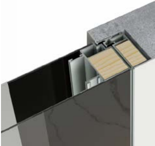
Короб прямого открывания RX 900, 93 мм
