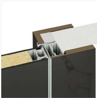
Полотно прямого открывания, толщина полотна 45 мм
