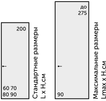
Короб реверсивного открывания R
