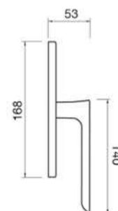
LE BOAT W2 Maniglia per finestra Window handle
