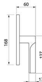
FIORD W2 Maniglia per finestra Window handle
