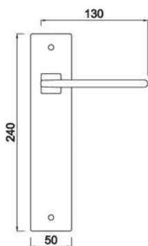
SPUTNIK PL Maniglia su rosetta placca Door lever handle with plate
