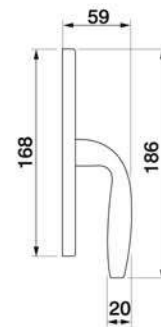
SIENA W2 Maniglia per finestra Window handle
