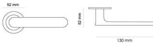
LE BOAT HM R1 Maniglia su rosetta con bocchetta Door lever handle with rosette and escutcheon
