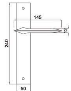
GALACTIC PL 2 Maniglia su rosetta placca Door lever handle with plate
