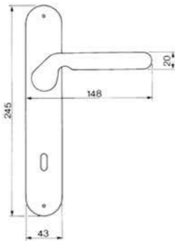
NIRVANA PL Maniglia su rosetta placca Door lever handle with plate
