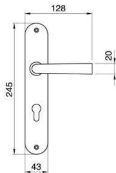
IDRO PL Maniglia su rosetta placca Door lever handle with plate
