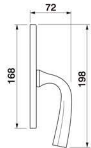
DREAM W2 Maniglia per finestra Window handle
