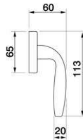
SIENA W1 Maniglia per finestra D.K. Window handle D.K.
