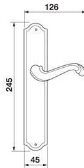
BAROCCO PL Maniglia su rosetta placca Door lever handle with plate
