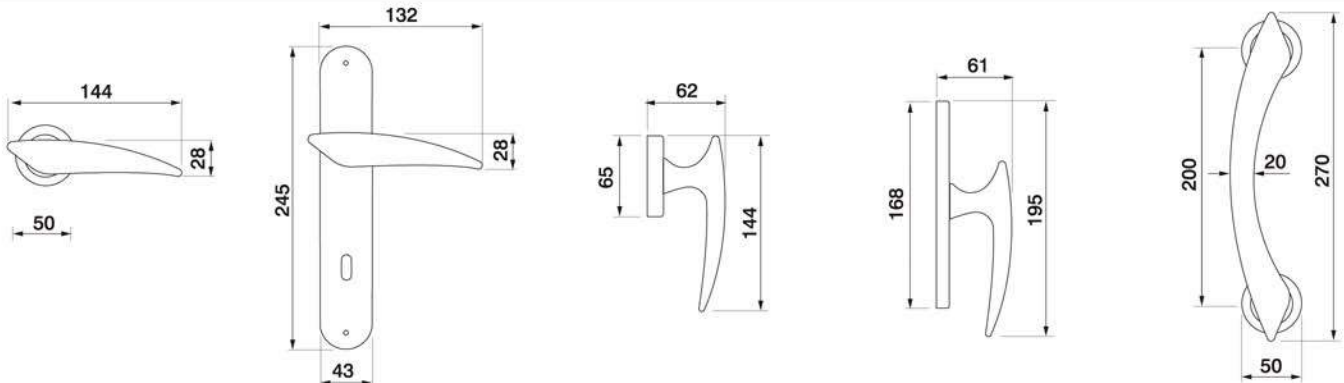
BOLID R2 Maniglia su rosetta con bocchetta Door lever handle with rosette and escutcheon
