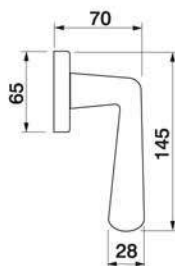
COCKATTO W1 Maniglia per finestra D.K. Window handle D.K.
