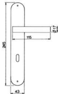
CALLA PL Maniglia su rosetta placca Door lever handle with plate
