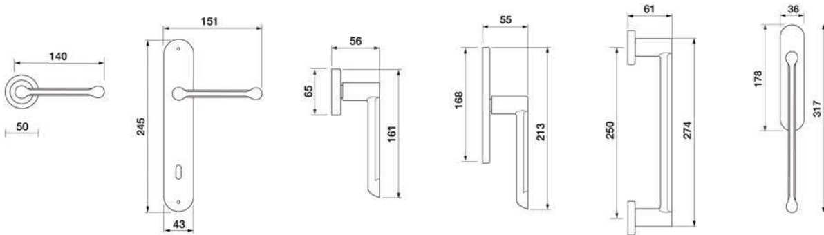
RAIN R2 Maniglia su rosetta con bocchetta Door lever handle with rosette and escutcheon
