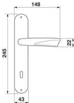
RAFT PL Maniglia su rosetta placca Door lever handle with plate
