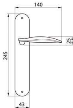
WAVE PL Maniglia su rosetta placca Door lever handle with plate
