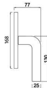
SPUTNIK W2 Maniglia per finestra Window handle
