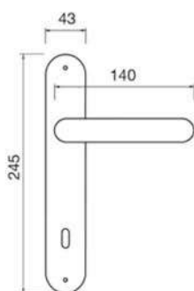
LE BOAT PL Maniglia su rosetta placca Door lever handle with plate
