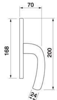
SAND W2 Maniglia per finestra Window handle
