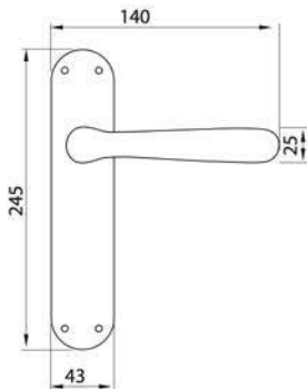
RUBINO PLB Maniglia su placca Door lever handle with plate
