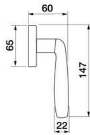
VENERA W1 Maniglia per finestra D.K. Window handle D.K.
