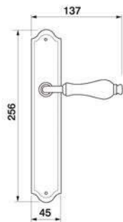
CERAMICA PL Maniglia su rosetta placca Door lever handle with plate
