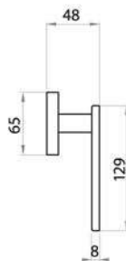
SPACE W1 Maniglia per finestra D.K. Window handle D.K.
