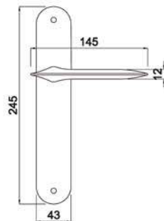
GALACTIC PL 1 Maniglia su rosetta placca Door lever handle with plate
