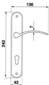
COBRA PL Maniglia su rosetta placca Door lever handle with plate
