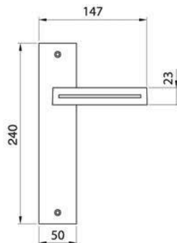
DIADEMA PL Maniglia su rosetta placca Door lever handle with plate
