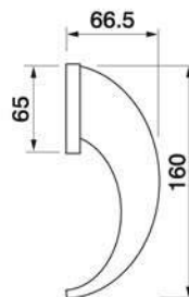
ABUNDANCE W1 Maniglia per finestra D.K. Window handle D.K.
