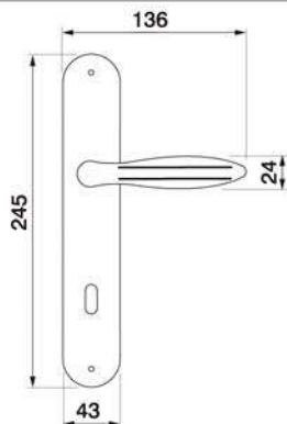
BUD PL Maniglia su rosetta placca Door lever handle with plate
