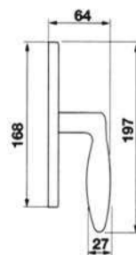
DALI W2 Maniglia per finestra Window handle
