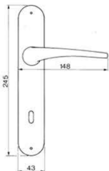
LE MANS PL Maniglia su rosetta placca Door lever handle with plate
