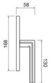
HARMONY W2 Maniglia per finestra Window handle
