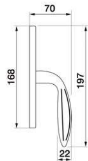
BUD W2 Maniglia per finestra Window handle
