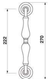
CERAMICA PH Maniglia Pull handle
