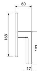
CULLINAN W2 Maniglia per finestra Window handle
