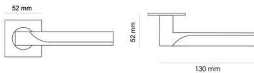
PLATEAU HM S2 Maniglia su rosetta con bocchetta Door lever handle with rosette and escutcheon
