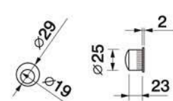
Set di serratura placche incasso con chiave complete di trascinatore Set of sliding door plate with flush pull, lock and key
