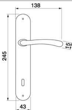
COCKATTO PL Maniglia su rosetta placca Door lever handle with plate
