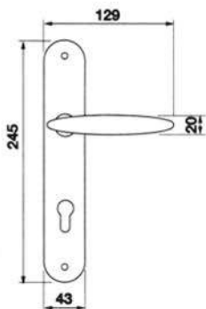
FLAMINGO PL Maniglia su rosetta placca Door lever handle with plate
