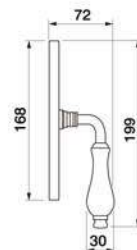
CERAMICA W2 Maniglia per finestra Window handle
