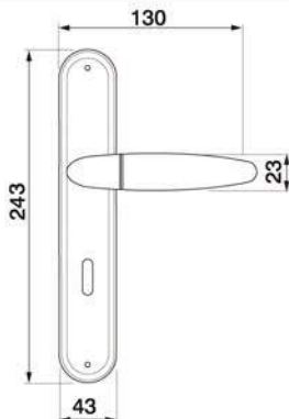
SAIL PL Maniglia su rosetta placca Door lever handle with plate
