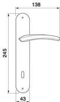
WIND PL Maniglia su rosetta placca Door lever handle with plate
