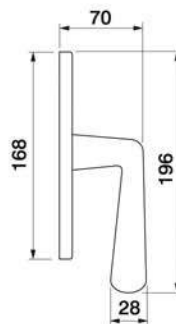
COCKATTO W2 Maniglia per finestra Window handle
