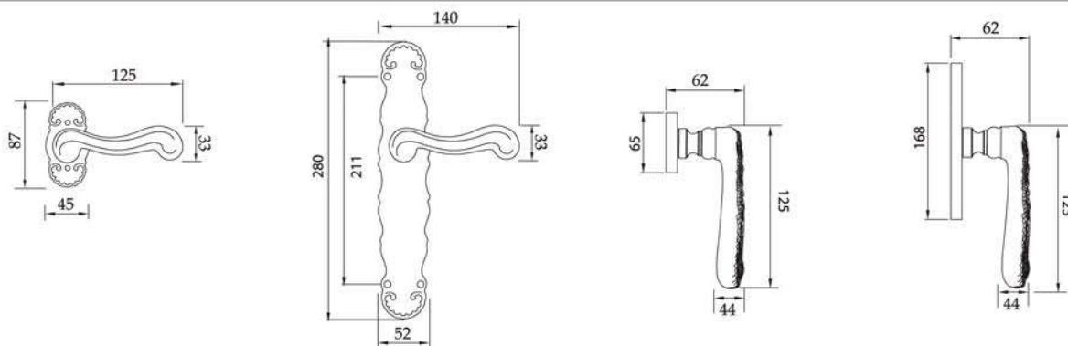
LOUVRE V Maniglia su rosetta con bocchetta Door lever handle with rosette and escutcheon
