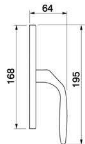
DERBY W2 Maniglia per finestra Window handle
