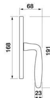
FRANCY W2 Maniglia per finestra Window handle
