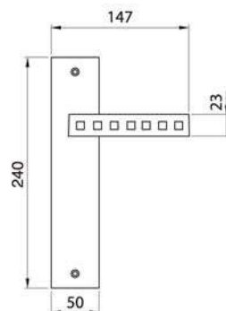
CULLINAN PL Maniglia su rosetta placca Door lever handle with plate
