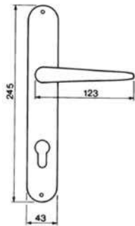
PETRA PL Maniglia su rosetta placca Door lever handle with plate
