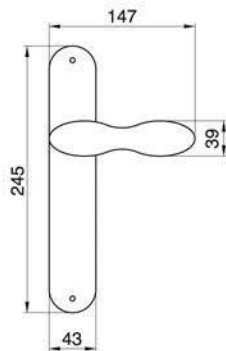
LUNCH PL Maniglia su rosetta placca Door lever handle with plate
