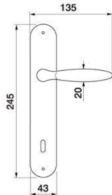
DERBY PL Maniglia su rosetta placca Door lever handle with plate
