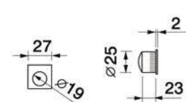
Set di serratura placche incasso con chiave complete di trascinatore Set of sliding door plate with flush pull, lock and key
