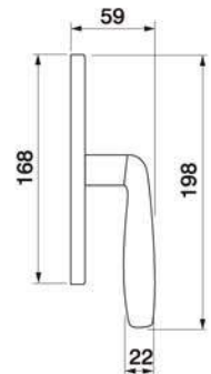
VENERA W2 Maniglia per finestra Window handle
