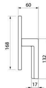
DDOLCE VITA W2 Maniglia per finestra Window handle
