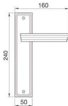
ALLURE PL Maniglia su rosetta placca Door lever handle with plate
