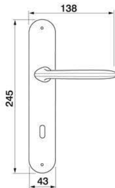
SAND PL Maniglia su rosetta placca Door lever handle with plate
