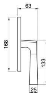
HILL W2 Maniglia per finestra Window handle
