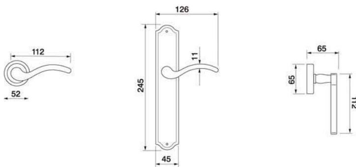
PATRICIA R2 Maniglia su rosetta con bocchetta Door lever handle with rosette and escutcheon
