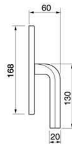
TENDER W2 Maniglia per finestra Window handle
