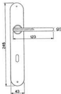
VERONICA PL Maniglia su rosetta placca Door lever handle with plate
