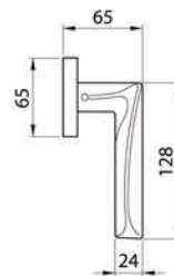
WAVE W1 Maniglia per finestra D.K. Window handle D.K.
