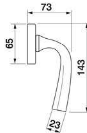
DREAM W1 Maniglia per finestra D.K. Window handle D.K.
