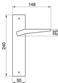
HILL PL Maniglia su rosetta placca Door lever handle with plate
