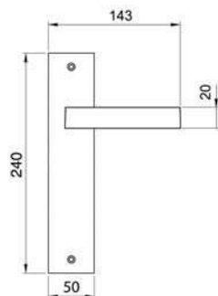
FIORD PL Maniglia su rosetta placca Door lever handle with plate
