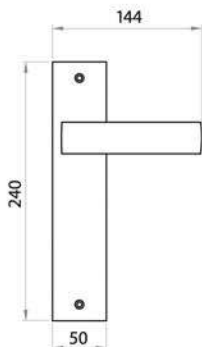
SPACE PL Maniglia su rosetta placca Door lever handle with plate
