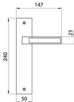
DDOLCE VITA PL Maniglia su rosetta placca Door lever handle with plate
