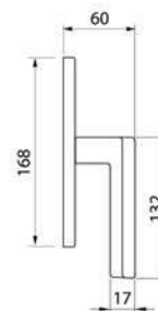
WATERFALL W2 Maniglia per finestra Window handle
