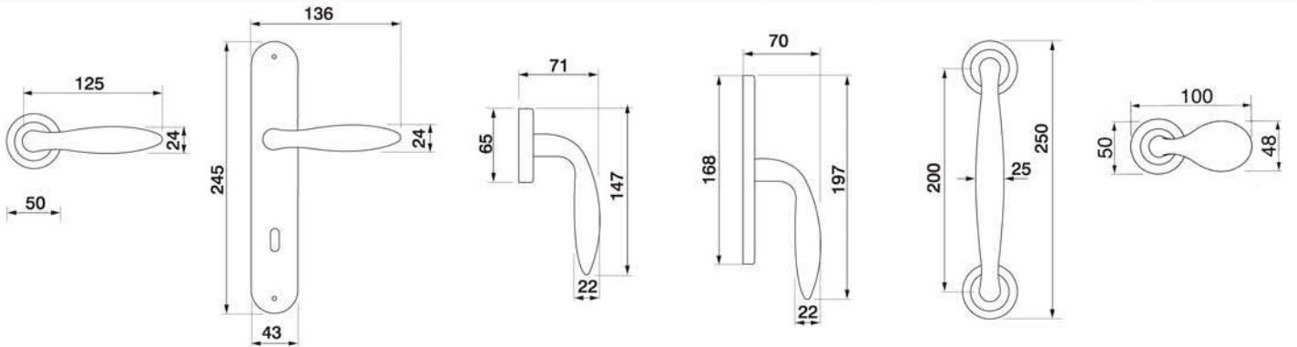
AIR R2 Maniglia su rosetta con bocchetta Door lever handle with rosette and escutcheon
