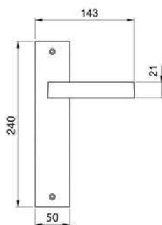
HORIZONTAL PL Maniglia su rosetta placca Door lever handle with plate
