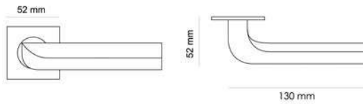
BRILLIANCE HM S2 Maniglia su rosetta con bocchetta Door lever handle with rosette and escutcheon
