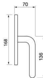
ALLURE W2 Maniglia per finestra Window handle
