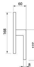
HORIZONTAL W2 Maniglia per finestra Window handle
