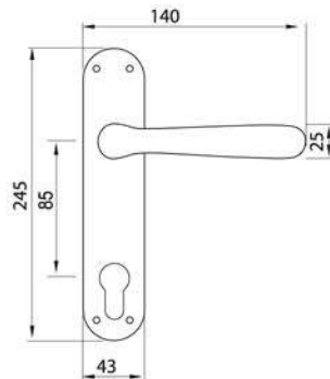
RUBINO PLB L85 Maniglia su rosetta placca Door lever handle with plate
