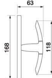
SAIL W2 Maniglia per finestra Window handle
