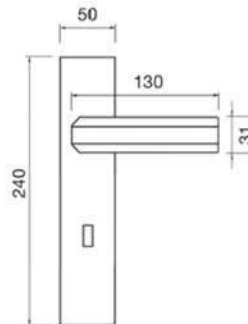
HARMONY PL Maniglia su rosetta placca Door lever handle with plate
