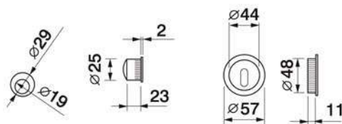
Set di serratura placche incasso con chiave complete di trascinatore Set of sliding door rose with flush pull, lock and key
