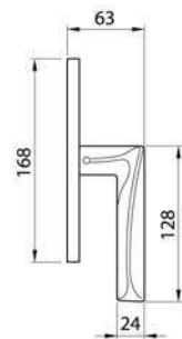
WAVE W2 Maniglia per finestra Window handle
