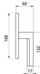
DIADEMA W2 Maniglia per finestra Window handle
