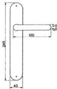
IRIS PL Maniglia su rosetta placca Door lever handle with plate
