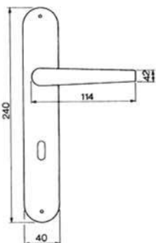
LILLA PL Maniglia su rosetta placca Door lever handle with plate
