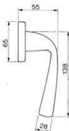
LE MANS W1 Maniglia per finestra D.K. Window handle D.K.
