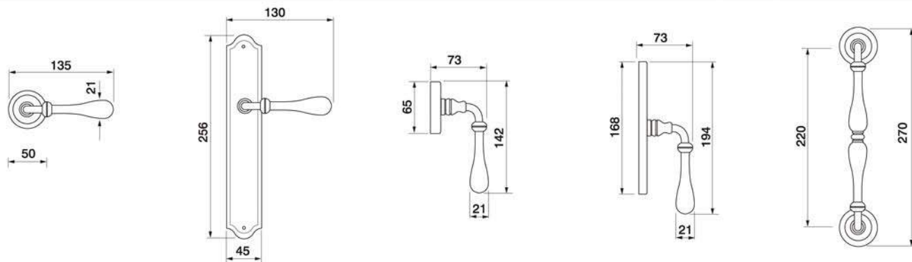
MARY R4 Maniglia su rosetta con bocchetta Door lever handle with rosette and escutcheon
