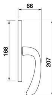
GOLF W2 Maniglia per finestra Window handle
