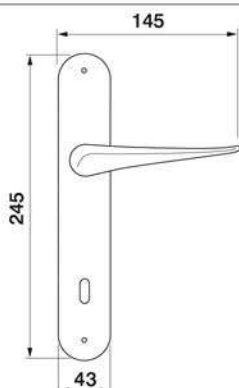
GOLF PL Maniglia su rosetta placca Door lever handle with plate
