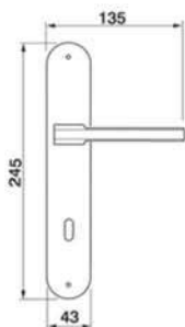
ROCK PL Maniglia su rosetta placca Door lever handle with plate
