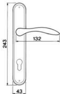
LEON PL Maniglia su rosetta placca Door lever handle with plate
