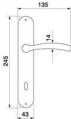
VENERA PL Maniglia su rosetta placca Door lever handle with plate
