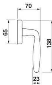
FRANCY W1 Maniglia per finestra D.K. Window handle D.K.
