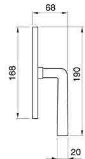
IDRO W2 Maniglia per finestra Window handle
