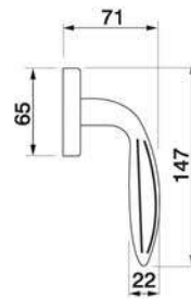
BUD W1 Maniglia per finestra D.K. Window handle D.K.
