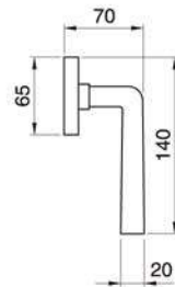
IDRO W1 Maniglia per finestra D.K. Window handle D.K.
