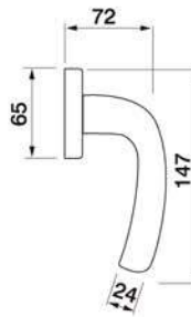
SAND W1 Maniglia per finestra D.K. Window handle D.K.
