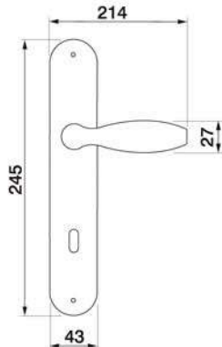
SIENA PL Maniglia su rosetta placca Door lever handle with plate
