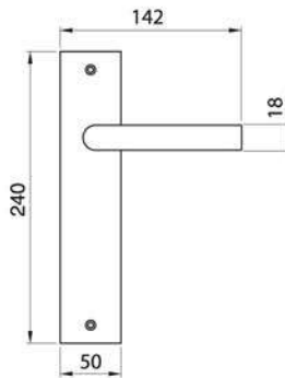
VOSTOK1 PL Maniglia su rosetta placca Door lever handle with plate
