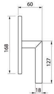
VOSTOK1 W2 Maniglia per finestra Window handle
