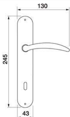
FRANCY PL Maniglia su rosetta placca Door lever handle with plate
