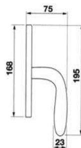
COBRA W2 Maniglia per finestra Window handle
