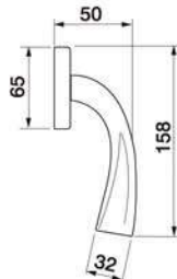
RAFT W1 Maniglia per finestra D.K. Window handle D.K.
