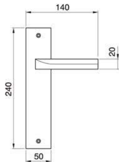
TENDER PL Maniglia su rosetta placca Door lever handle with plate
